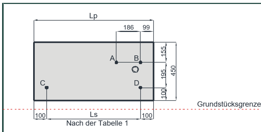
ZEICHNUNG 3 POSITIONIERUNG DER GEWINDESTANGEN. (am Beispiel eines Schiebetors mit Öffnungsrichtung LINKS (Ansicht von der Straße)
